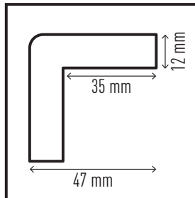
Profilo paracolpi angolare C35 #1102-130 - adesivo #1112-130 - magnetico
