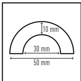
Profilo paracolpi per superfici tubolari P30 #1115-130
