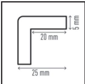
Profilo paracolpi angolare C20 #1101-130 - adesivo #1111-130 - magnetico
