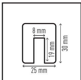
Profilo paracolpi per spigoli E8 #1127-130
