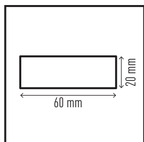
Profilo paracolpi per superfici piane S20 #1108-130
