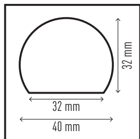
Profilo paracolpi per superfici piane S32R #1109-130
