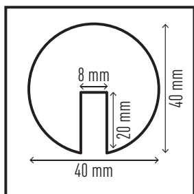
Profilo paracolpi per spigoli E8R #1126-130
