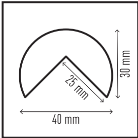
Profilo paracolpi angolare C25R #1100-130 - adesivo #1110-130 - magnetico
